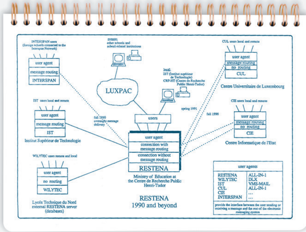
Schéma d'interconnexion du réseau RESTENA en 1990 // The RESTENA network's interconnection diagram in 1990
